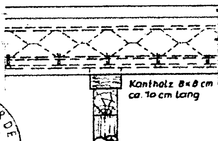
Montageunterstützung ohne Querrippe
