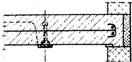
Endfeld 157cm in Vollbeton und Verankerung der Querrippe im Randbalken
