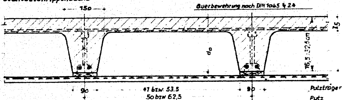
Stahlbetonrippendecke
