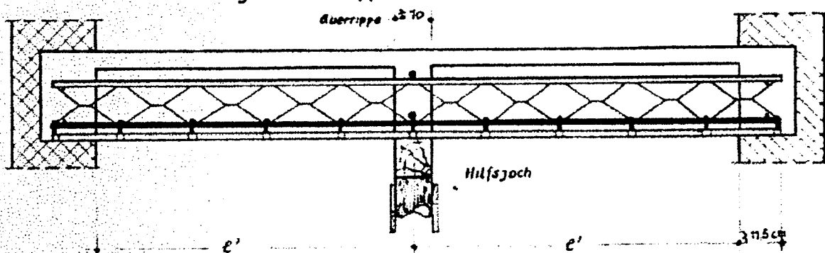
Ausbildung der Querrippen und Hilfsunterstützung
